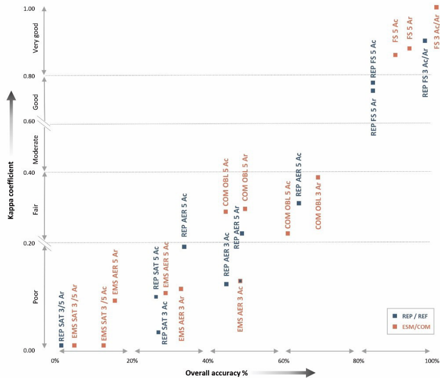
Figura 5. Análisis de la exactitud global y el coeficiente kappa según la fuente de datos y el número de categorías consideradas.
